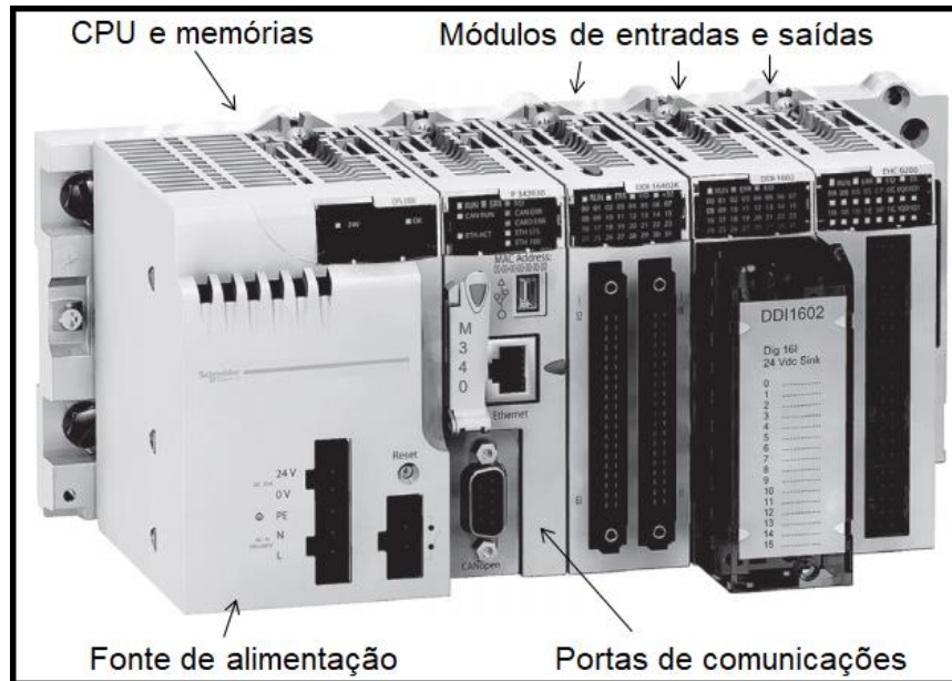
Figura 9. Controlador lógico programável. Fonte: Petruzella (2014) adaptado pelo autor.
