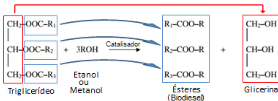
Figura 4. Processo de transesterificação do biodiesel. Fonte: CHIONG et al. (2018). Adaptado pelo autor.
