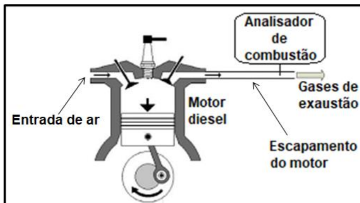
Figura 30. Sonda do analisador inserido no escapamento do motor.
