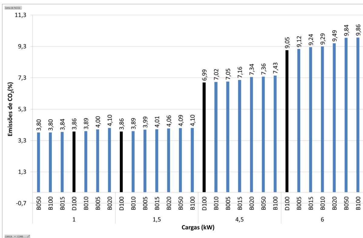
Figura 36. Emissões de dióxido de carbono para os combustíveis testados.
