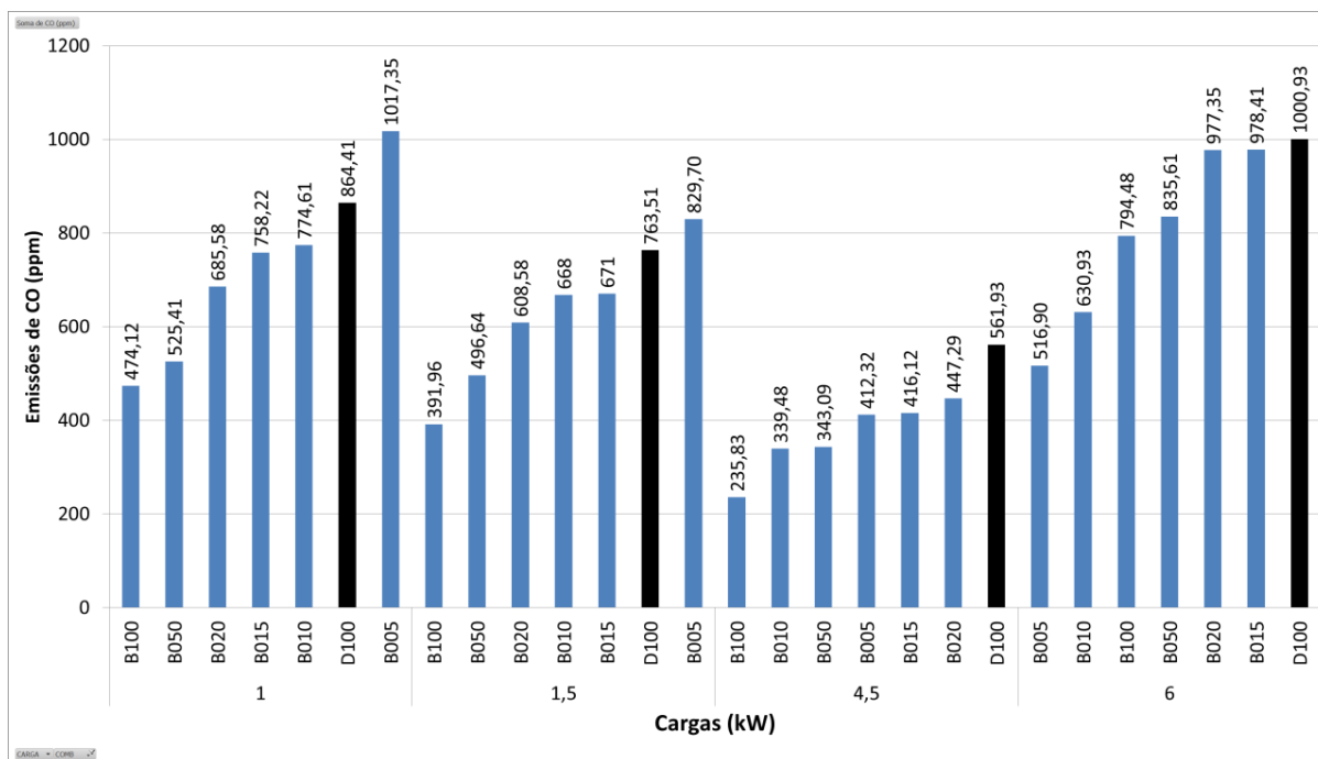
Figura 35. Emissões de monóxido de carbono para os combustíveis avaliados.
