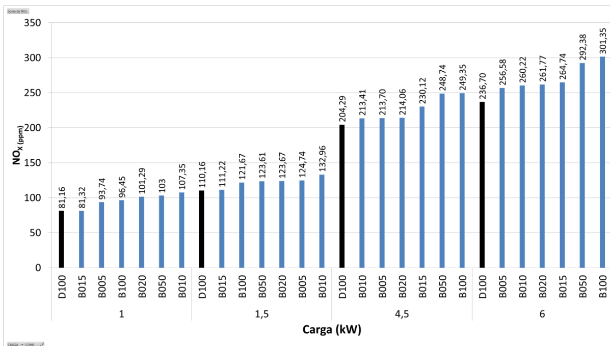
Figura 34. Emissões de NO x para os combustíveis avaliados nos estudos.
