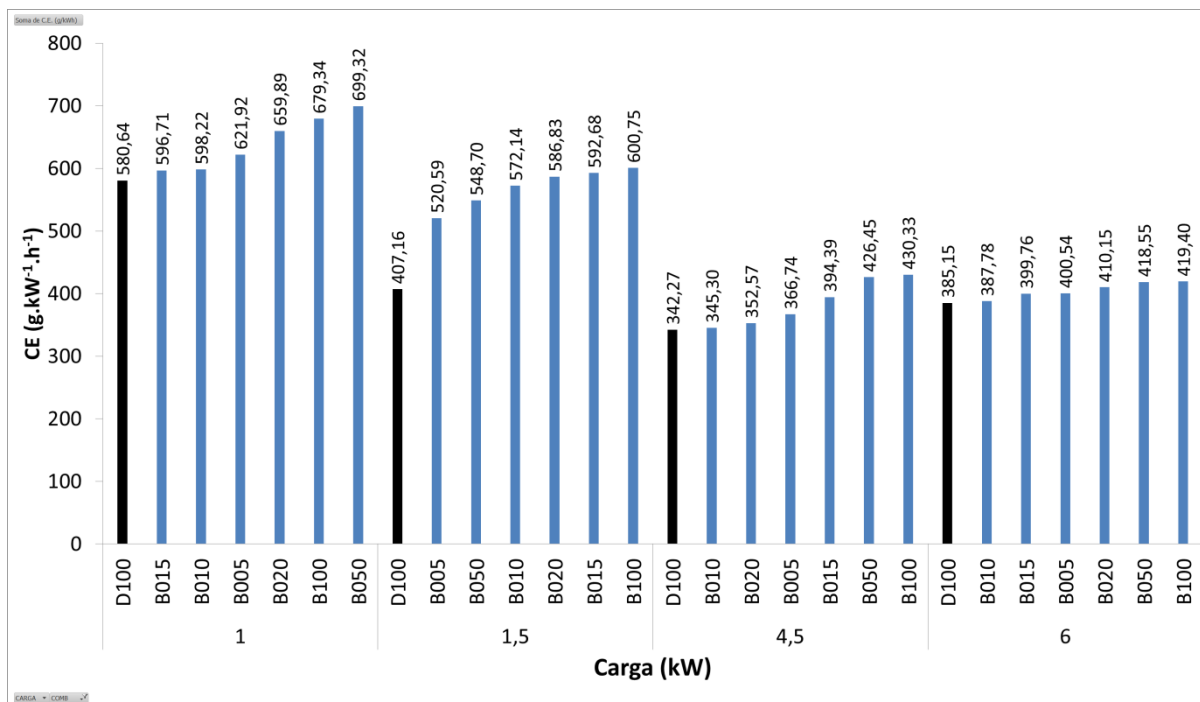
Figura 33. Consumo específico dos combustíveis para as cargas testados.
