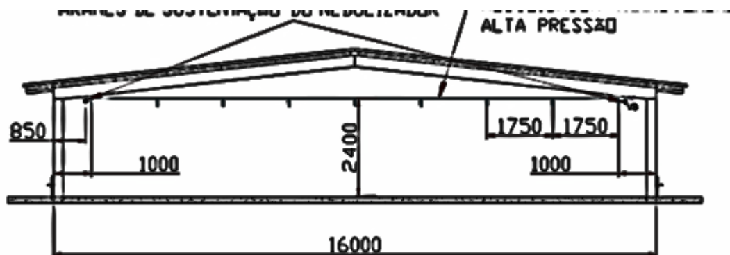
Figura 6: Croqui sistema de nebulização. Fonte: AGROMARAU GSI, 2017, adaptado pela autora.
