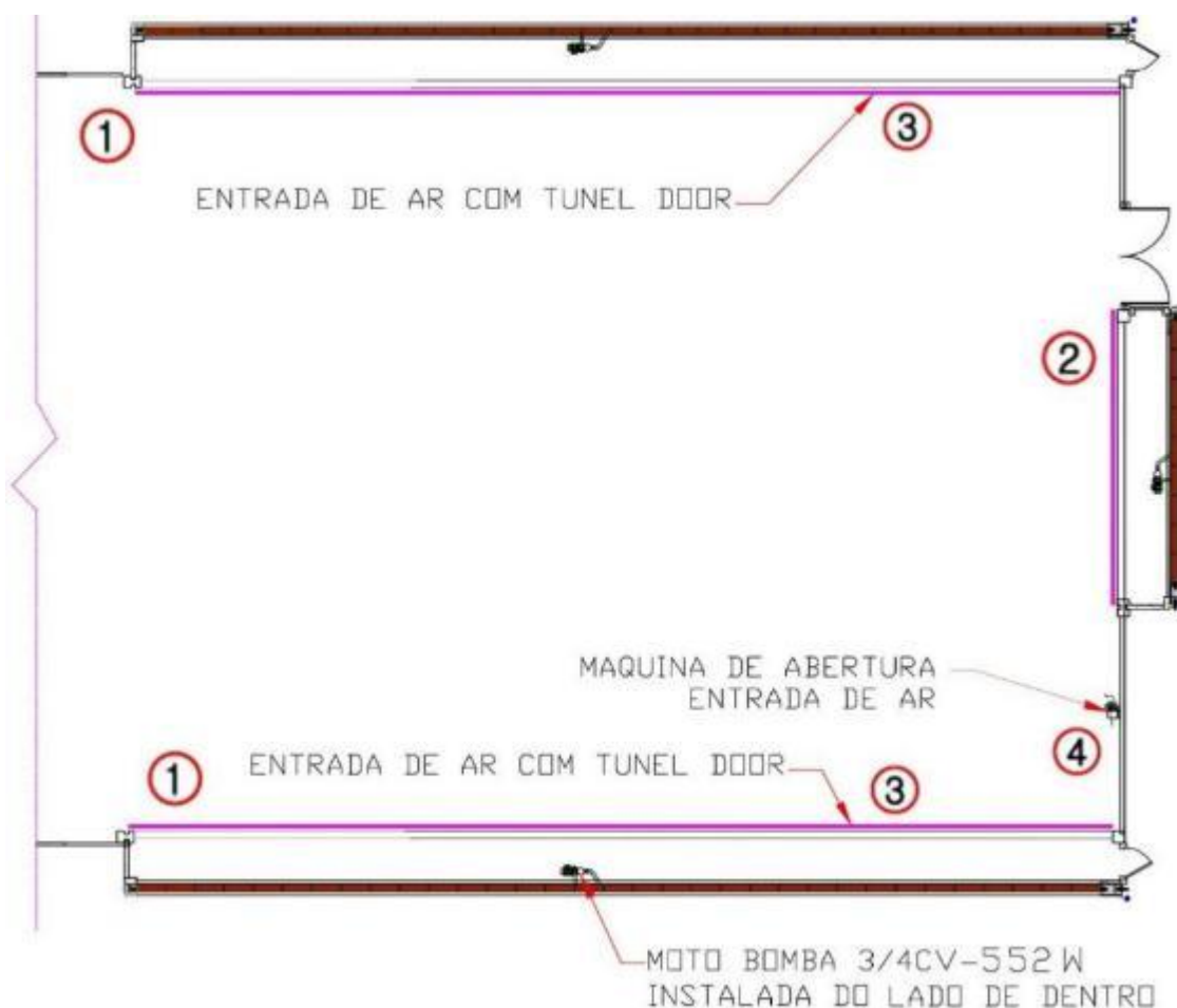
Figura 27: Sistema de resfriamento – Pad cooling . Croqui de distribuição. (1) Painéis evaporativos pad cooling ativos (2) Painel evaporativo pad cooling desativado (3) Sistema de ventilação túnel door (4) Máquina de abertura entrada de ar túnel door .
