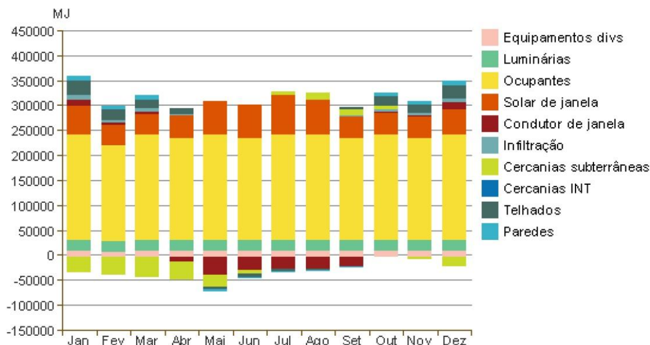
Gráfico 10: Carga mensal de resfriamento, aviário projeto proposto.
