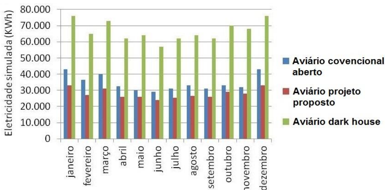
Gráfico 12: Consumo mensal de eletricidade simulada, nos três modelos de aviários comparados.
