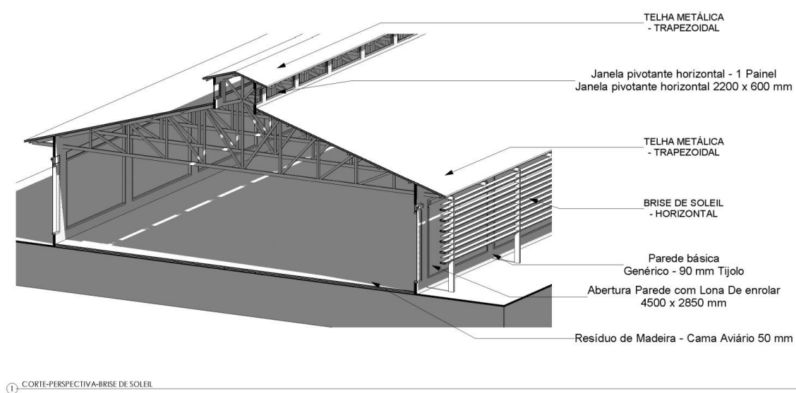
Figura 13: Projeto proposto. (corte perspectivado)
