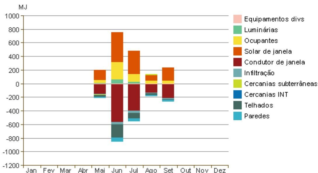
Gráfico 6: Carga mensal de aquecimento, aviário convencional aberto.
