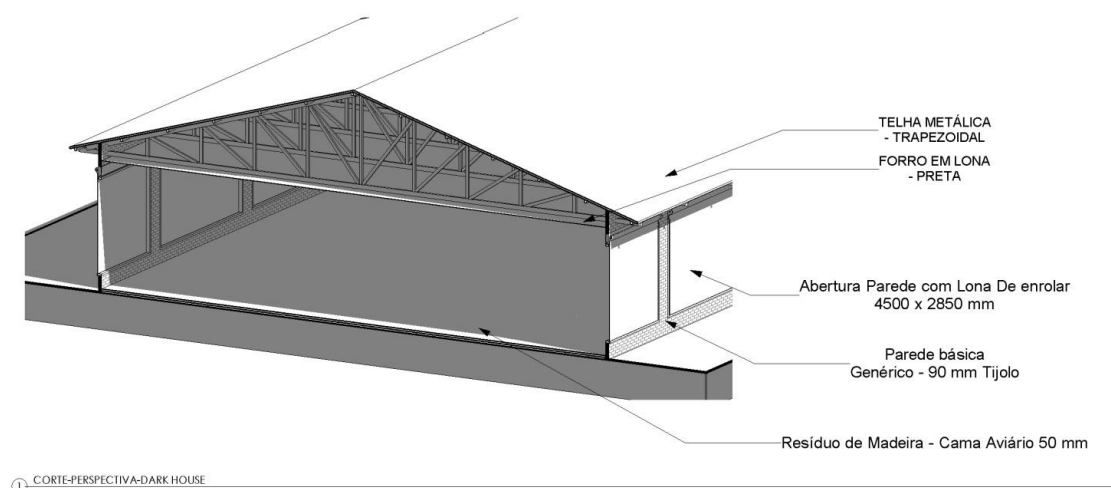
Figura 16: Sistema Dark House . (corte perspectivado)
