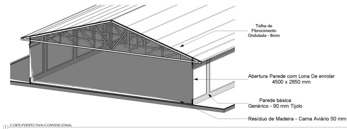
Figura 8: Sistema convencional aberto (corte perspectivado)
