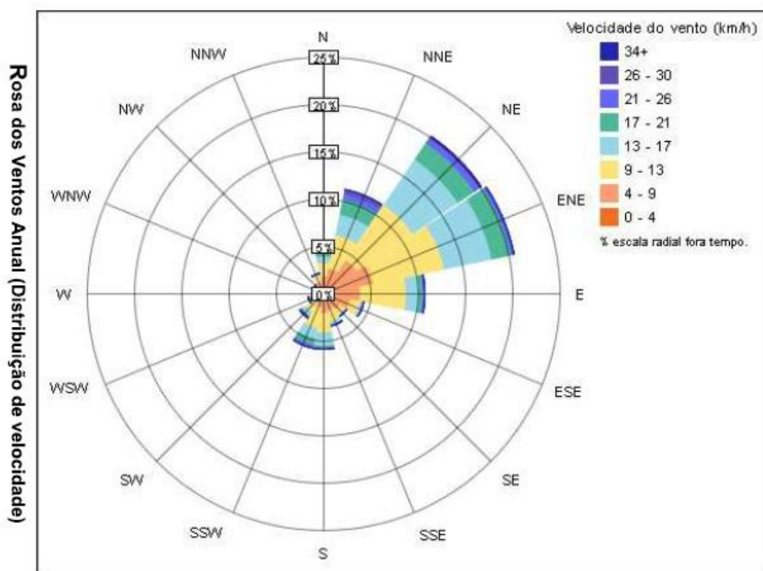
Figura 5: Velocidade e direção dos ventos na estação meteorológica, no local de implantação dos três modelos de aviários comparados.
