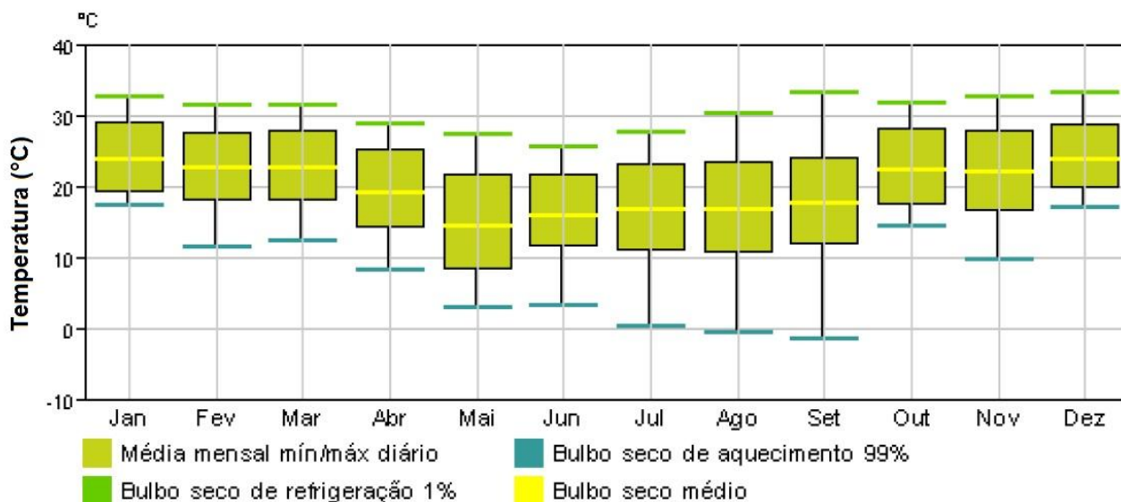
Gráfico 2: Dados mensais de bulbo seco, da estação meteorológica, no local de implantação dos três modelos de aviários comparados.
