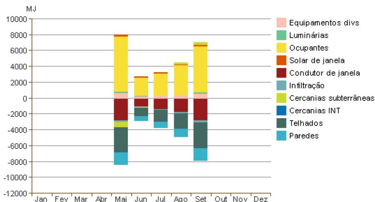
Gráfico 8: Carga mensal de aquecimento, aviário dark house.
