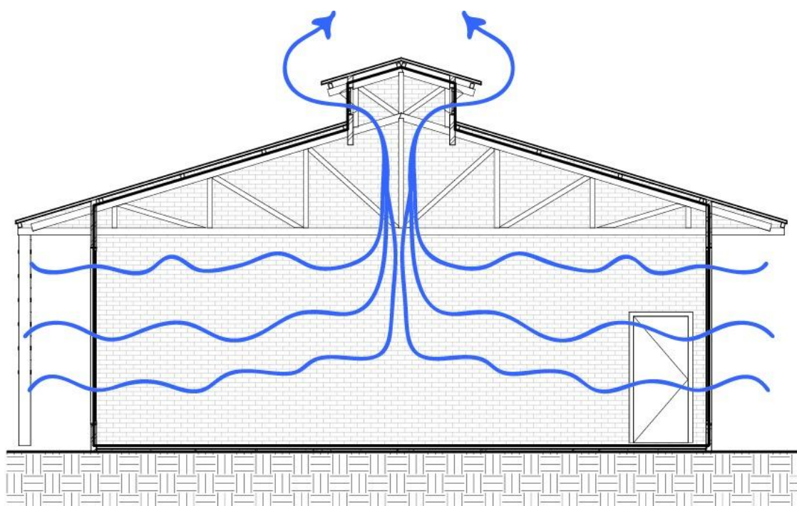
Figura 10: Efeito Chaminé
