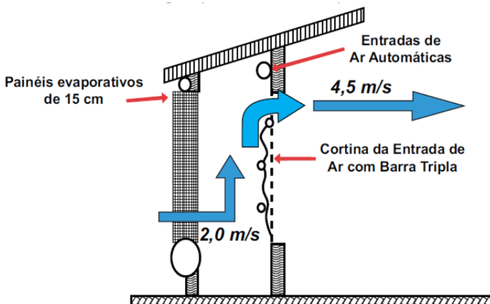
Figura 17: Detalhe sistema pad coolings, utilizado no aviário dark house . (Fonte: COBB-VANTRESS, 2008)
