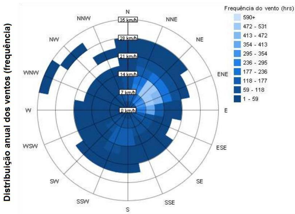
Figura 20: Frequência anual dos ventos da estação meteorológica, no local de implantação dos três modelos de aviários comparados .
