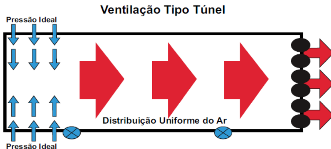
Figura 19: Sistema ventilação túnel de vento. (aviário dark house ) (Fonte: COBB-VANTRESS, 2008)
