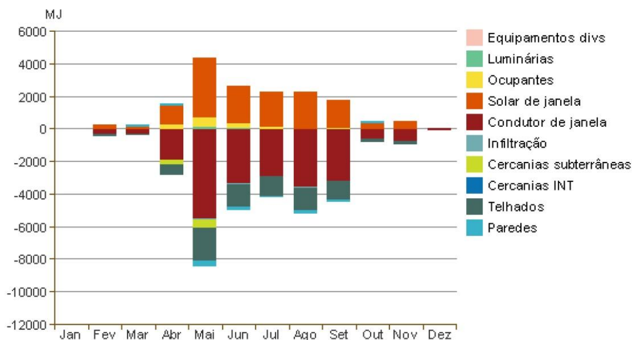
Gráfico 7: Carga mensal de aquecimento, aviário projeto proposto.
