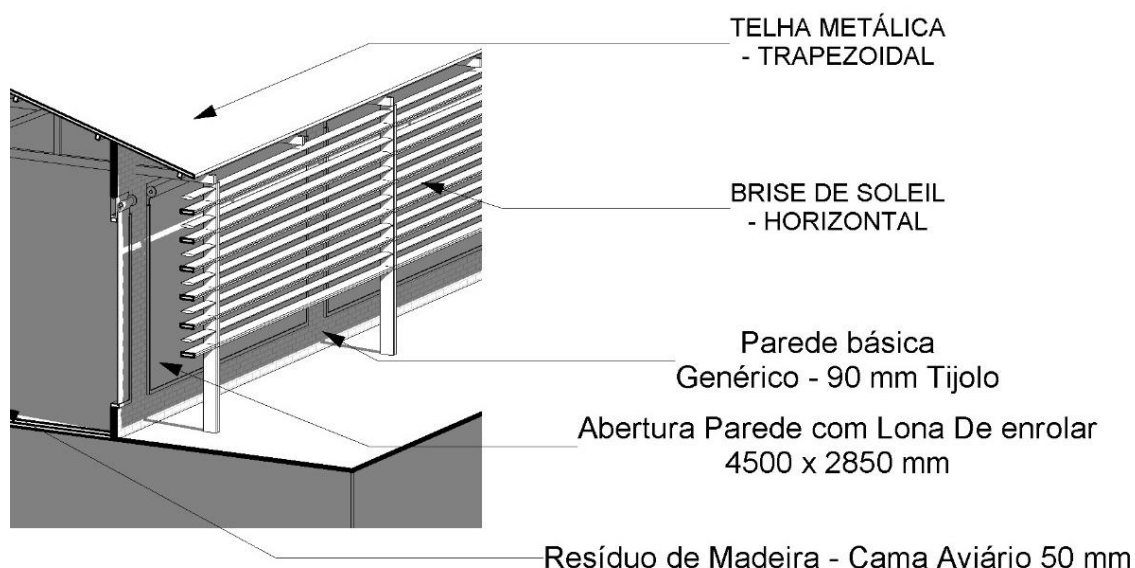
Figura 9: detalhe sistema de brises.
