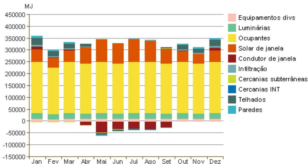
Gráfico 9: Carga mensal de resfriamento, aviário convencional aberto.
