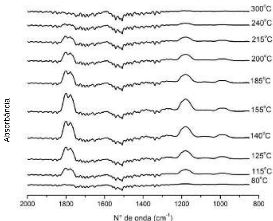
Figura 27: Espectro por infravermelho de gases removidos do processo de adsorção de ácido acético em fase de gás sobre H-Beta. Condições: Fluxo de N_2 20 mL min -1 , variação de temperatura de 50-600°C, com rampa de aquecimento de 10 °C/min.
