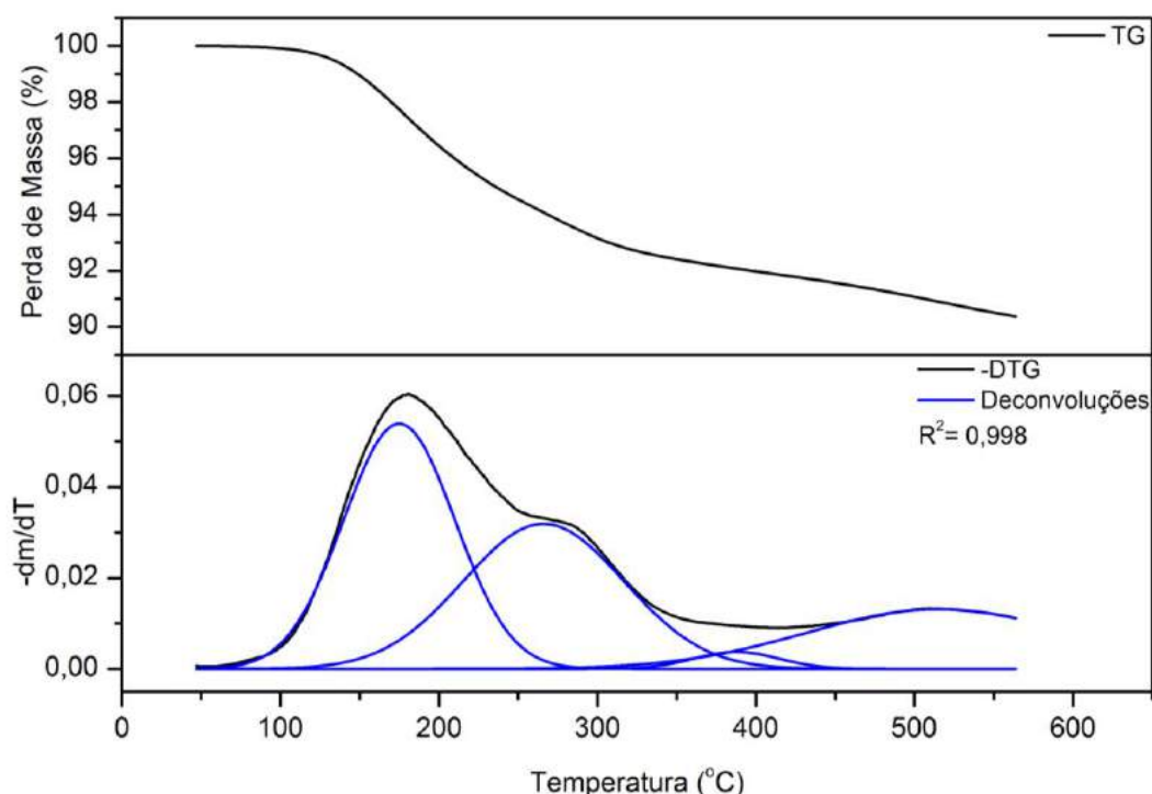
Figura 26: Termograma com TG, DTG e deconvolução para a remoção de ácido acético da superfície da zeólita H-Beta. Condições: Fluxo de N 2 20 mL min -1 , variação de temperatura de 50 até 565°C, com rampa de aquecimento de 10 °C/min.
