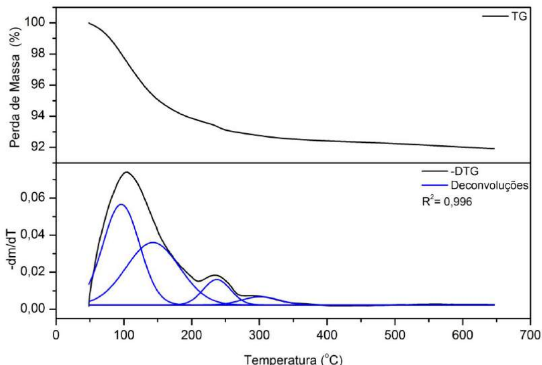
Figura 28: Termograma com TG, DTG e deconvolução para a remoção de metanol da superfície da zeólita H-Beta. Condições: Fluxo de N_2 20 mL min^{-1} , variação de temperatura de 50 até 650°C, com rampa de aquecimento de 10 °C/min.
